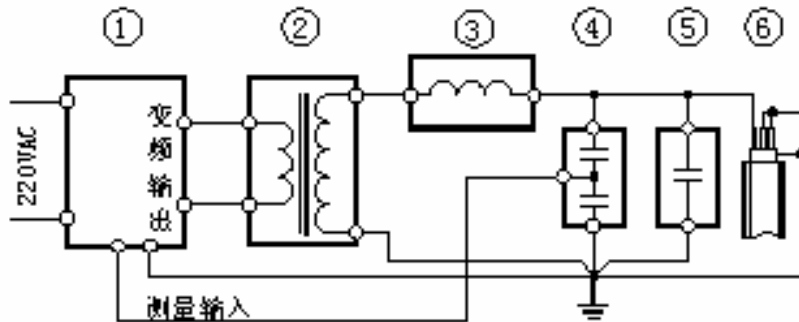
电缆耐压试验接线图A
