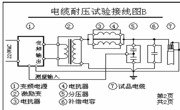
图. 3.4.1 用于测试电缆耐压的串联谐振接线图.
