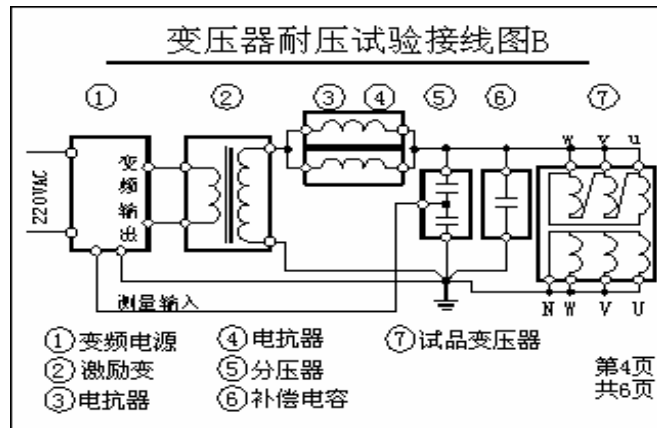
图. 3.4.2 用于测试变压器耐压的串联谐振接线图.
